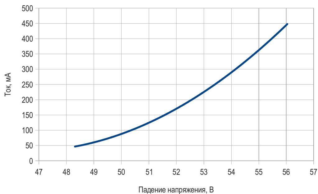
Вольт-амперная характеристика
