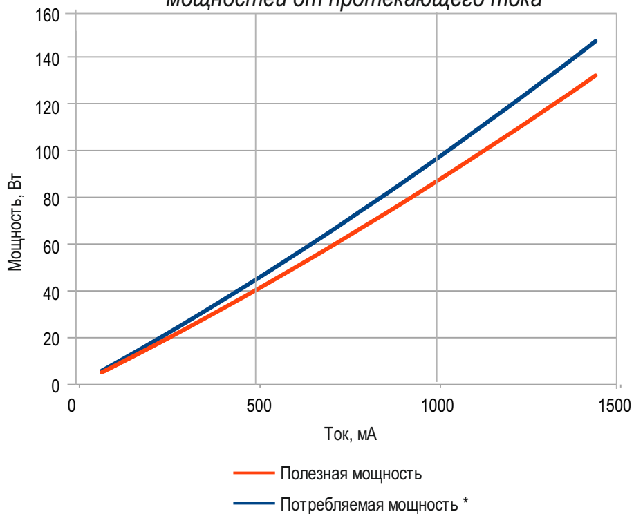
График зависимости полезной и потребляемой* мощностей от протекающего тока
