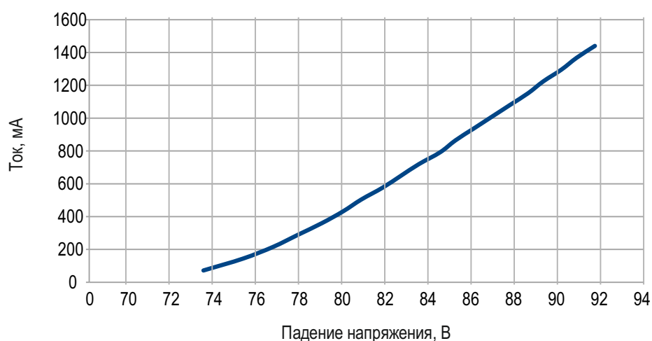
График зависимости падения напряжения от протекающего тока
