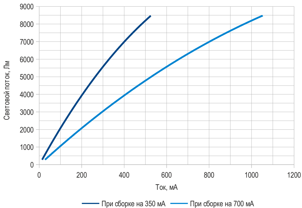
График зависимости светового потока от поданного тока
