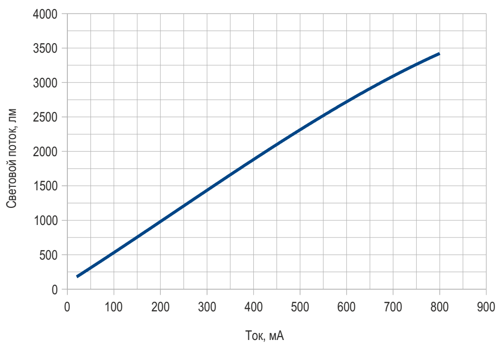
График зависимости светового потока от поданного тока
