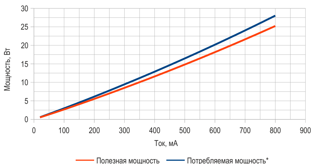
График зависимости полезной (потребляемой*) мощности от поданного тока
