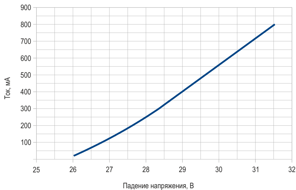
Вольт-амперная характеристика
