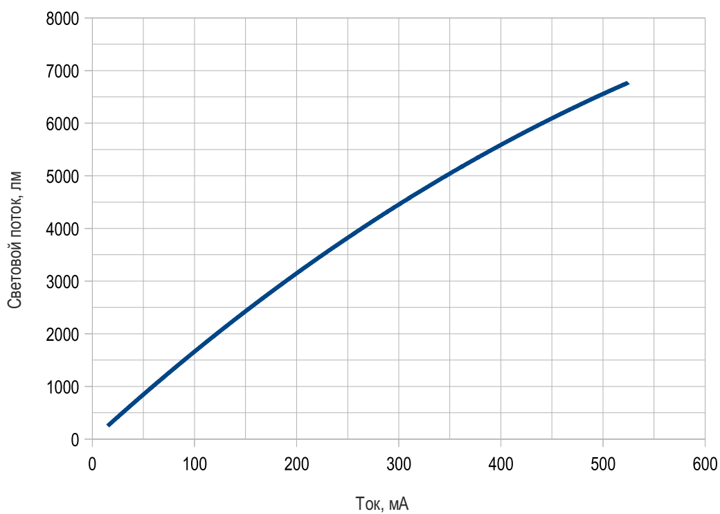
График зависимости светового потока от поданного тока
