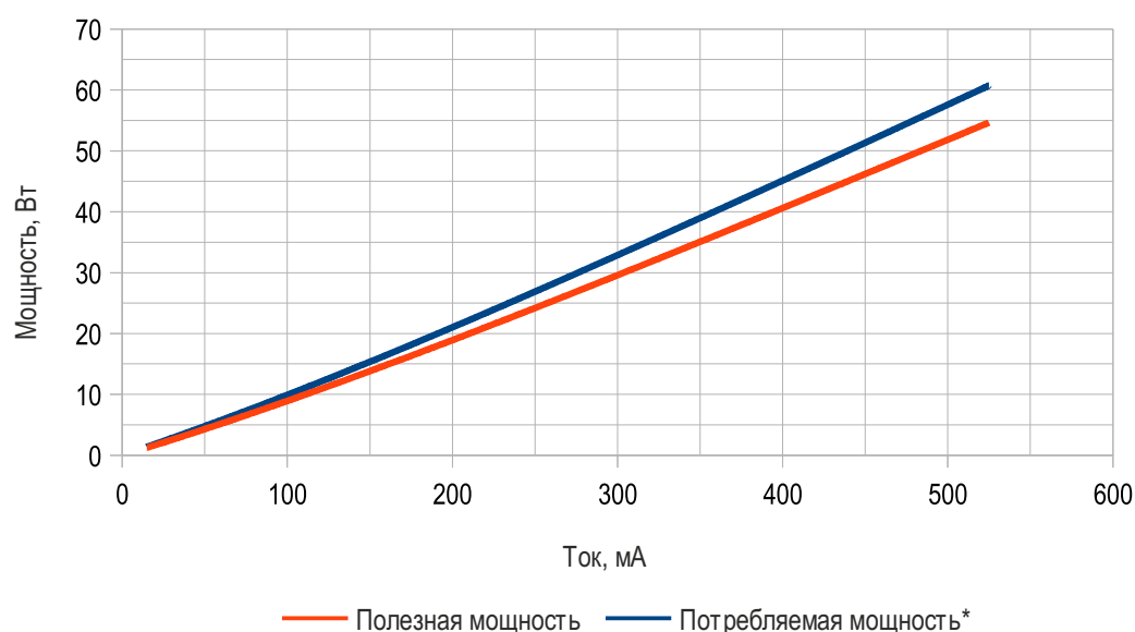
График зависимости полезной (потребляемой*) мощности от поданного тока
