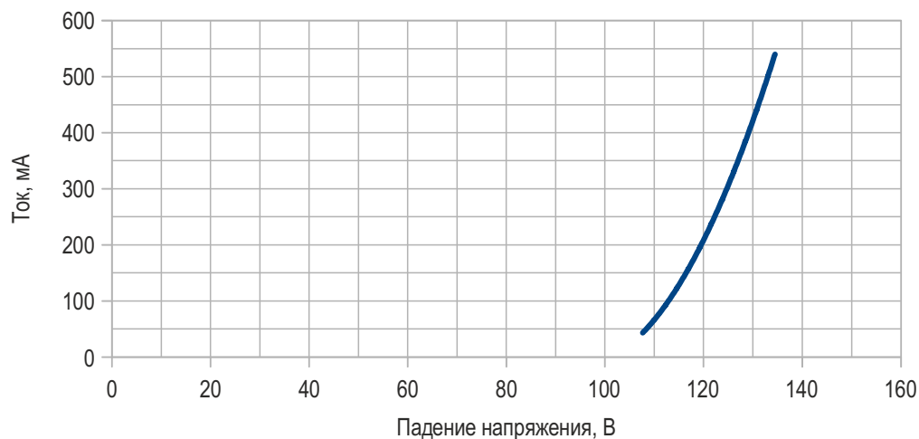
Вольт-амперная характеристика
