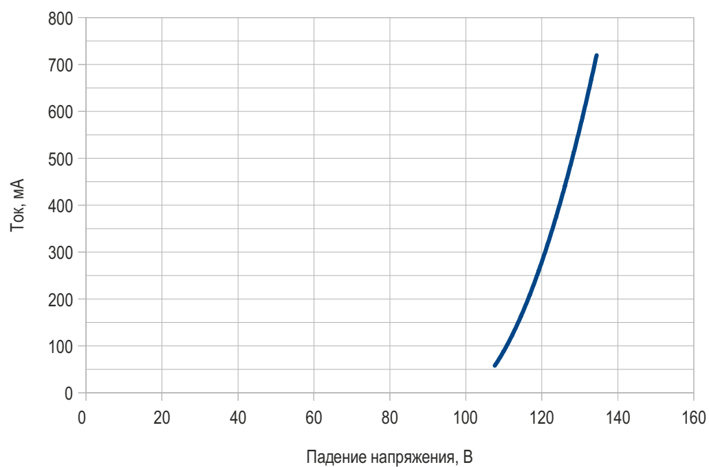
Вольт-амперная характеристика
