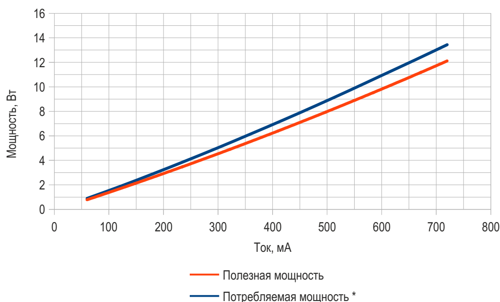
График зависимости полезной и потребляемой* мощностей от поданного тока
