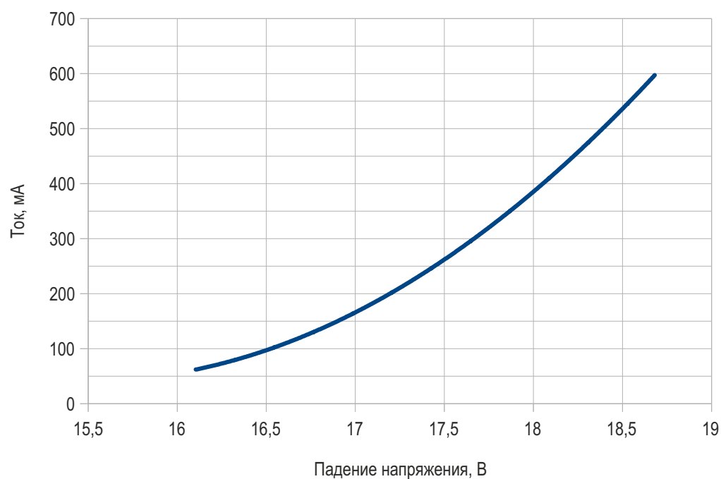
Вольт-амперная характеристика
