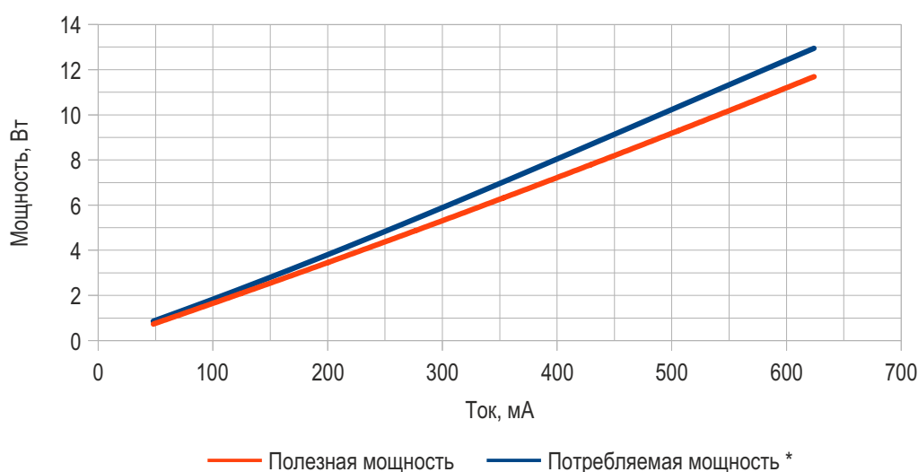
График зависимости полезной и потребляемой* мощностей от поданного тока
