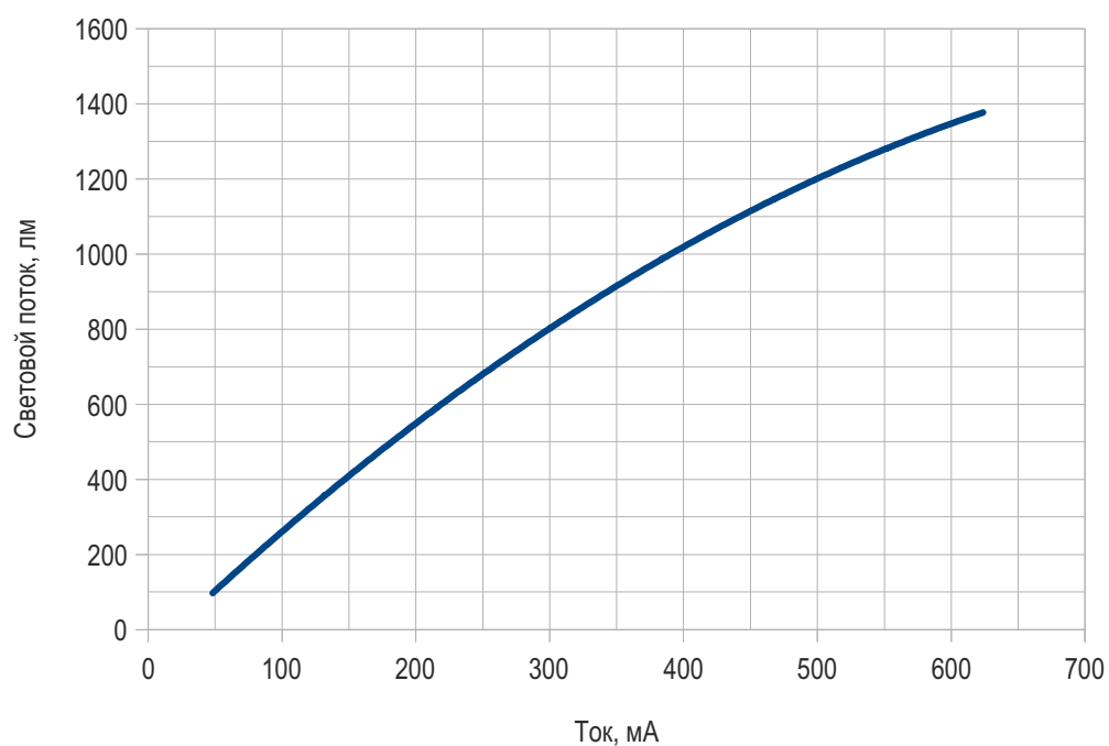
График зависимости светового потока от поданного тока
