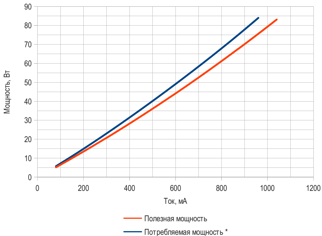
График зависимости полезной и потребляемой* мощностей от поданного тока
