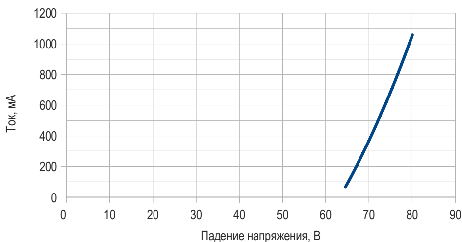
Вольт-амперная характеристика
