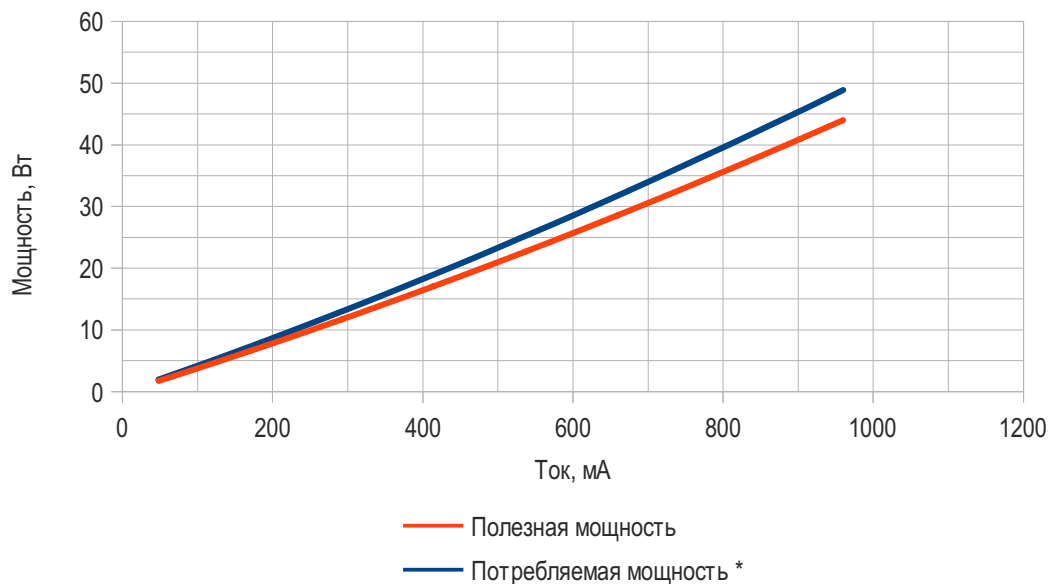
График зависимости полезной и потребляемой* мощностей от поданного тока
