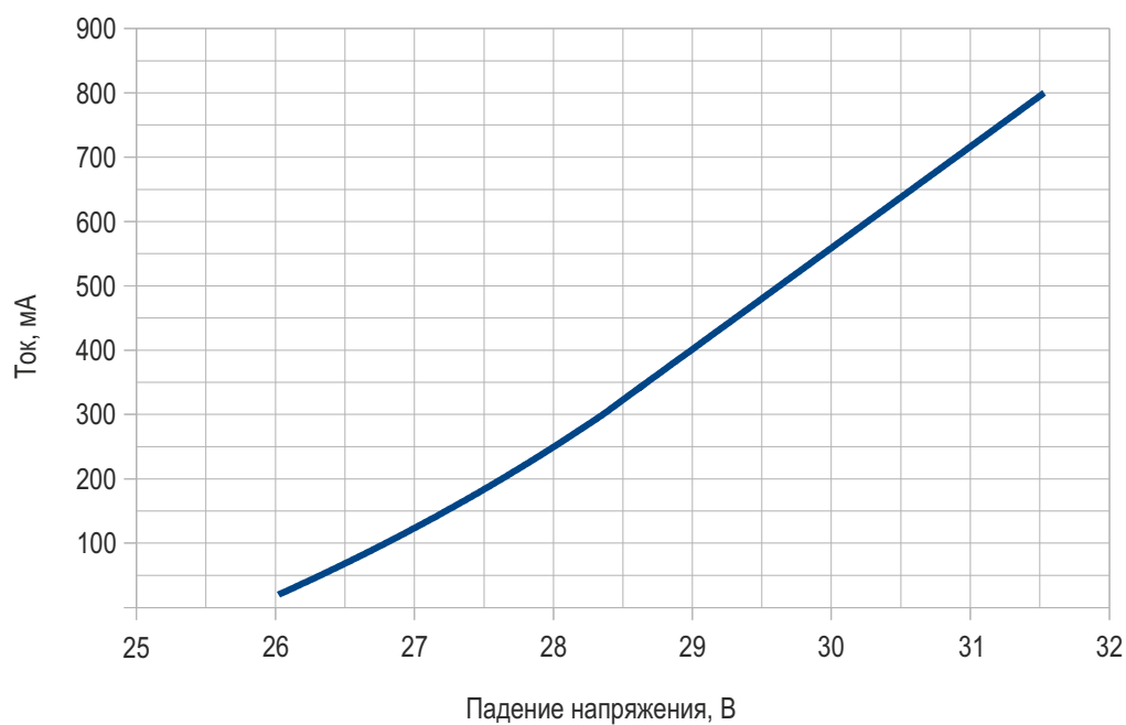
Вольт-амперная характеристика
